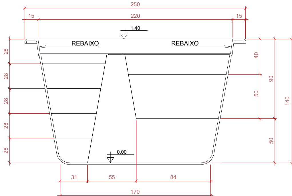
CORTE TRANSVERSAL SEM ESCALA
