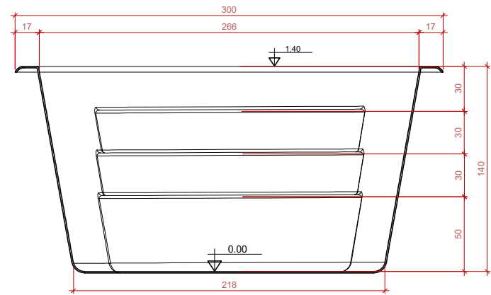
CORTE TRANSVERSAL SEM ESCALA
