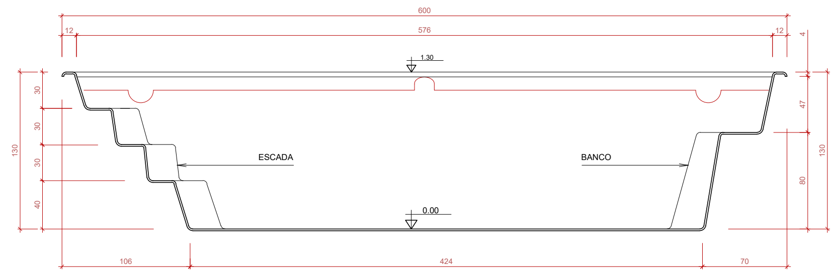
CORTE LONGITUDINAL SEM ESCALA
