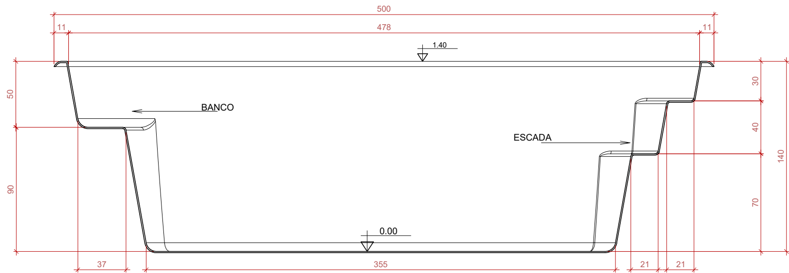
CORTE LONGITUDINAL SEM ESCALA
