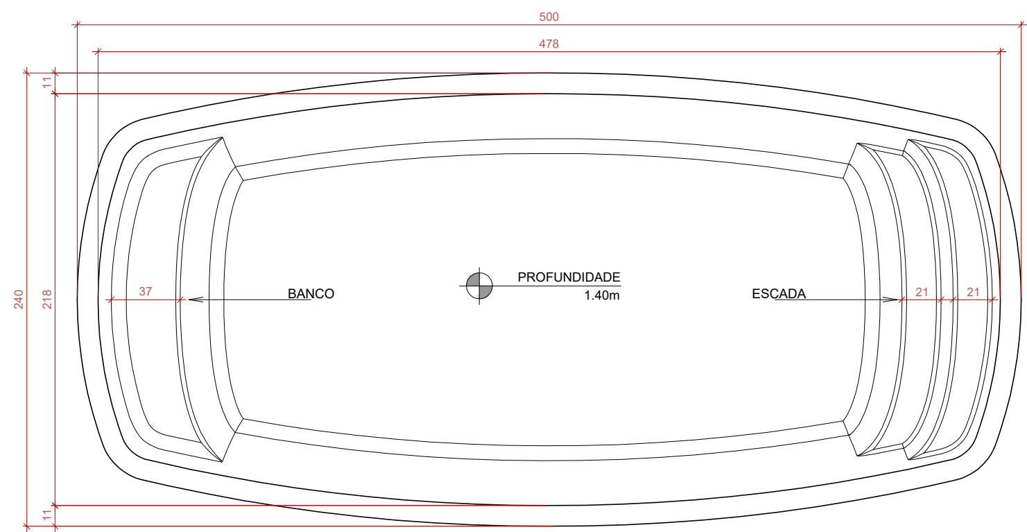
PLANTA BAIXA SEM ESCALA
