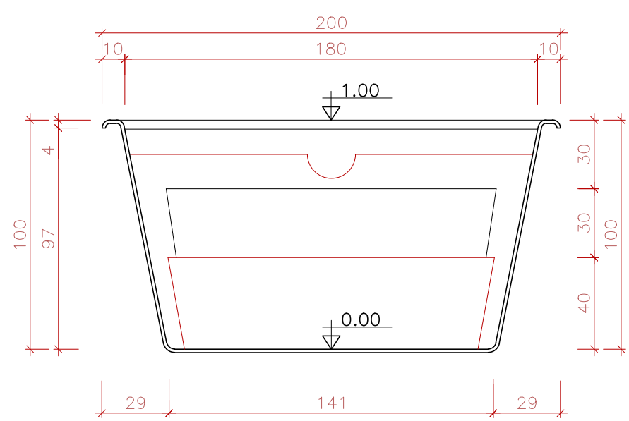
CORTE TRANSVERSAL SEM ESCALA
