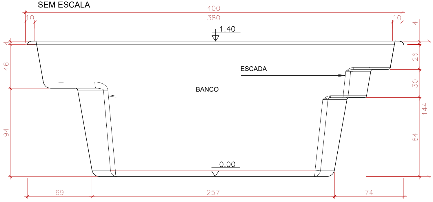
CORTE LONGITUDINAL SEM ESCALA
