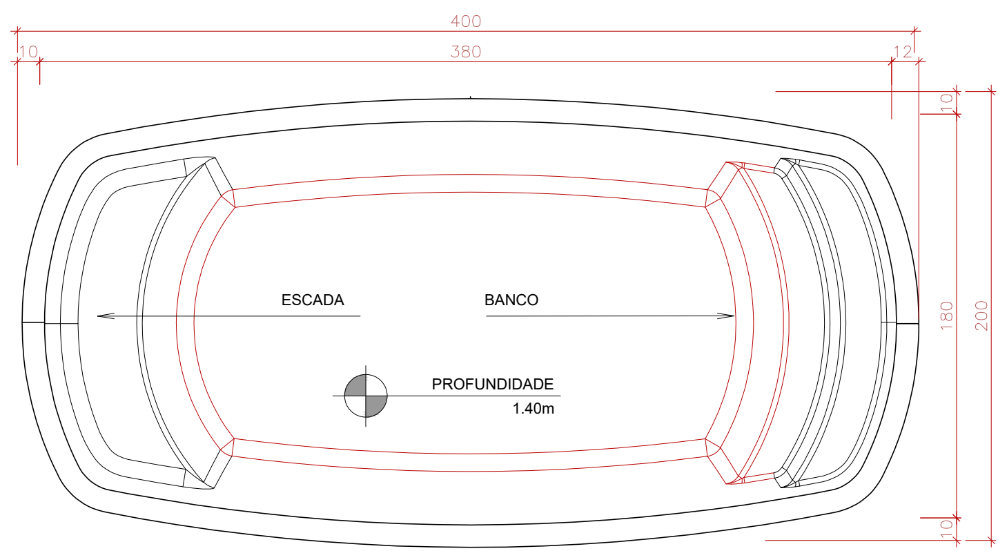
PLANTA BAIXA SEM ESCALA
