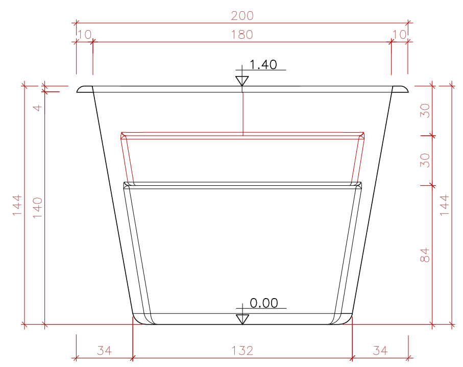
CORTE TRANSVERSAL SEM ESCALA
