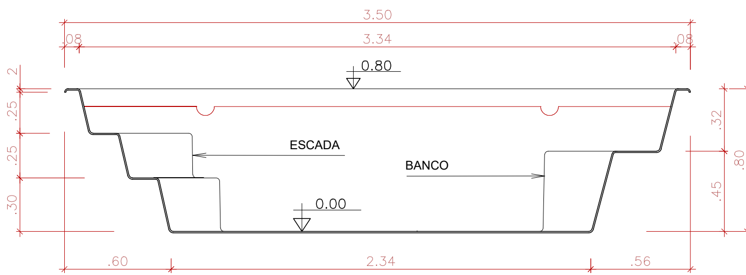
CORTE LONGITUDINAL SEM ESCALA
