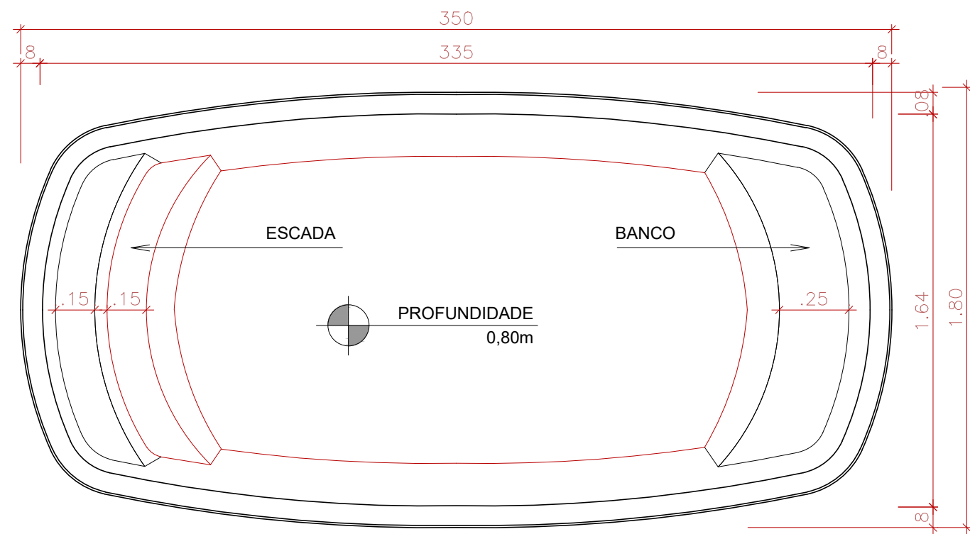
PLANTA BAIXA SEM ESCALA
