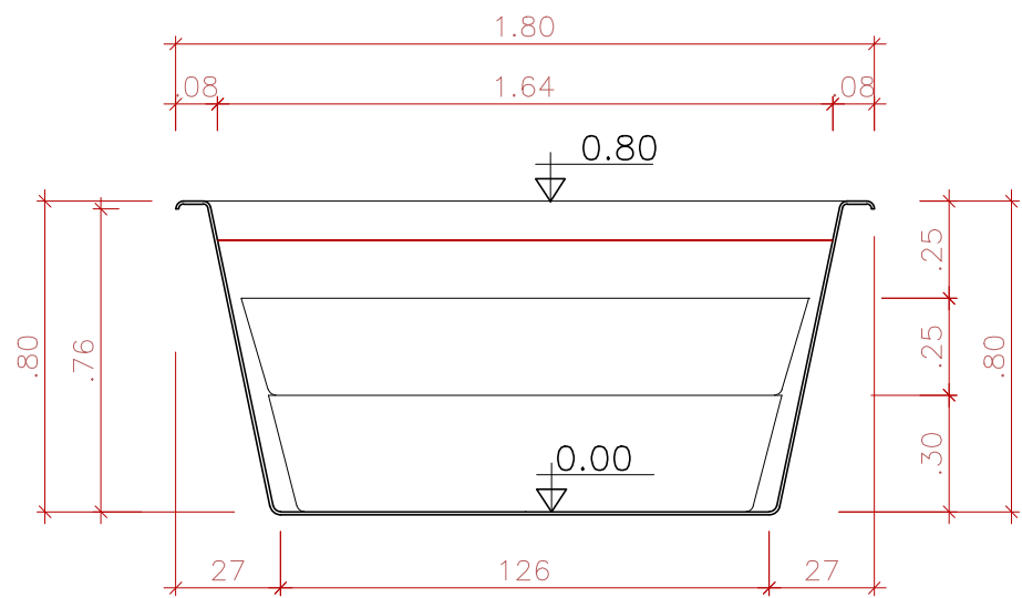
CORTE TRANSVERSAL SEM ESCALA
