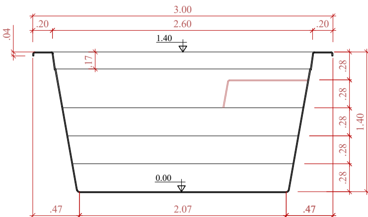
CORTE TRANSVERSAL SEM ESCALA
