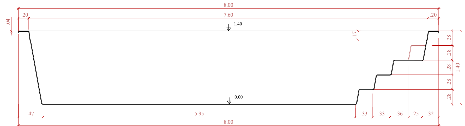
CORTE LONGITUDINAL SEM ESCALA
