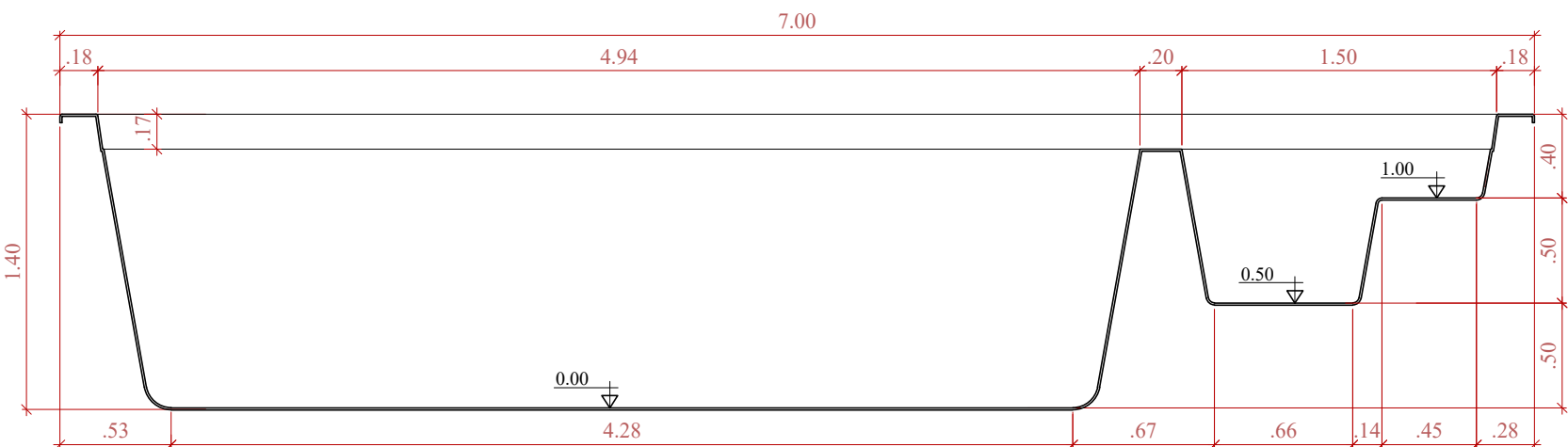
CORTE LONGITUDINAL SEM ESCALA
