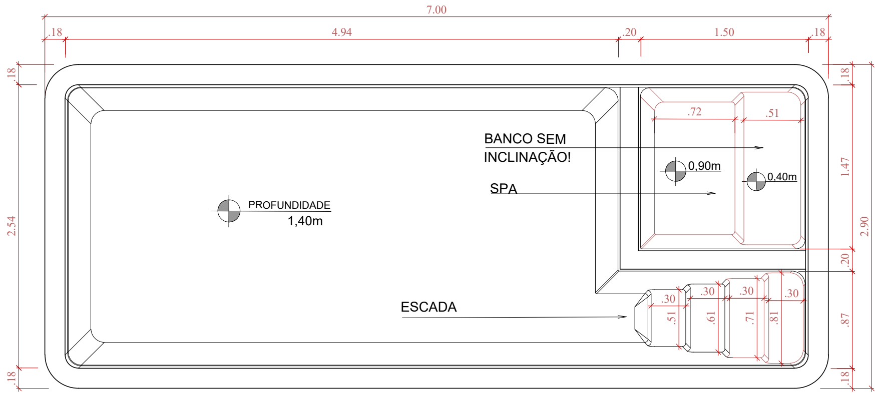
PLANTA SEM ESCALA
