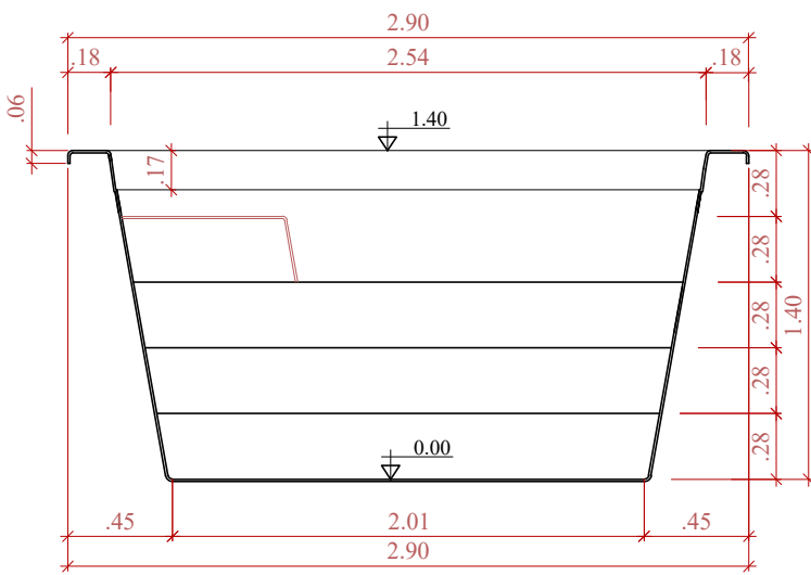
CORTE TRANSVERSAL SEM ESCALA
