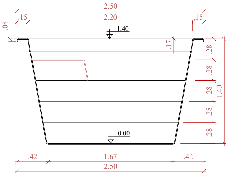
CORTE TRANSVERSAL SEM ESCALA
