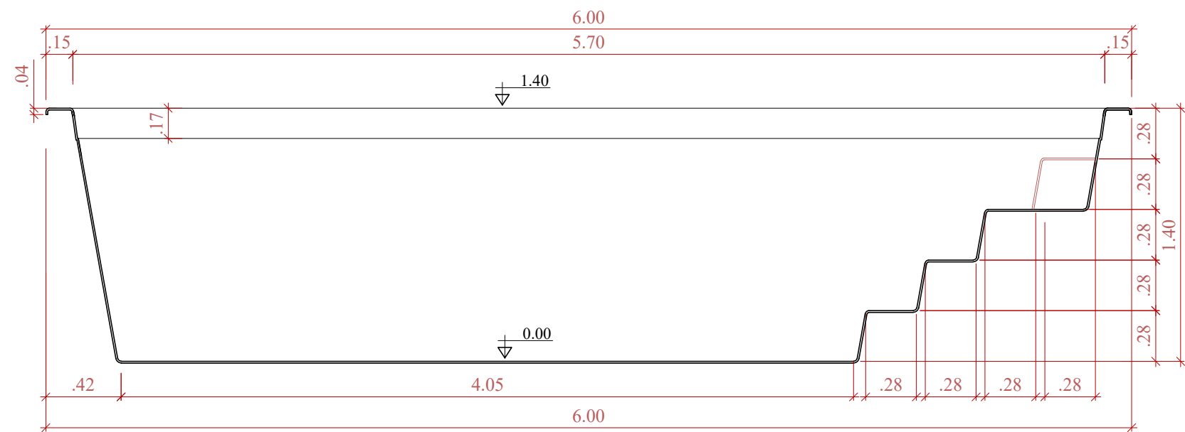
CORTE LONGITUDINAL SEM ESCALA
