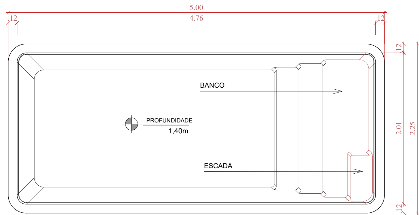
PLANTA SEM ESCALA
