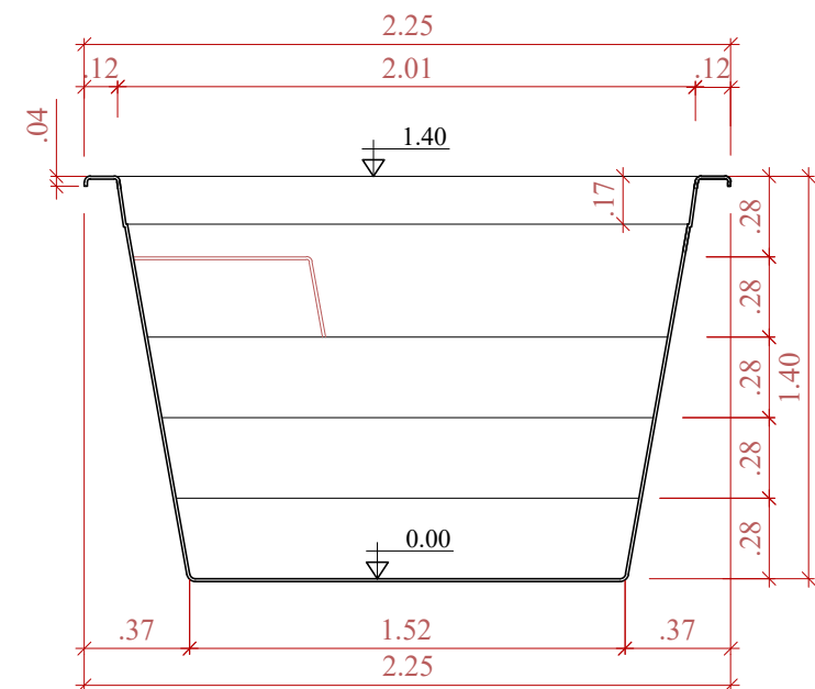
CORTE TRANSVERSAL SEM ESCALA
