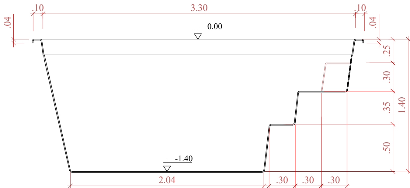
CORTE LONGITUDINAL SEM ESCALA
