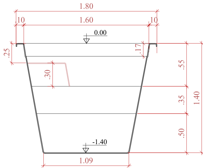
CORTE TRANSVERSAL SEM ESCALA
