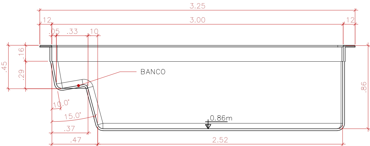
CORTE LONGITUDINAL SEM ESCALA
