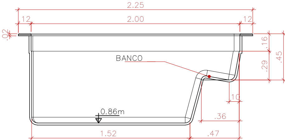
CORTE TRANSVERSAL SEM ESCALA
