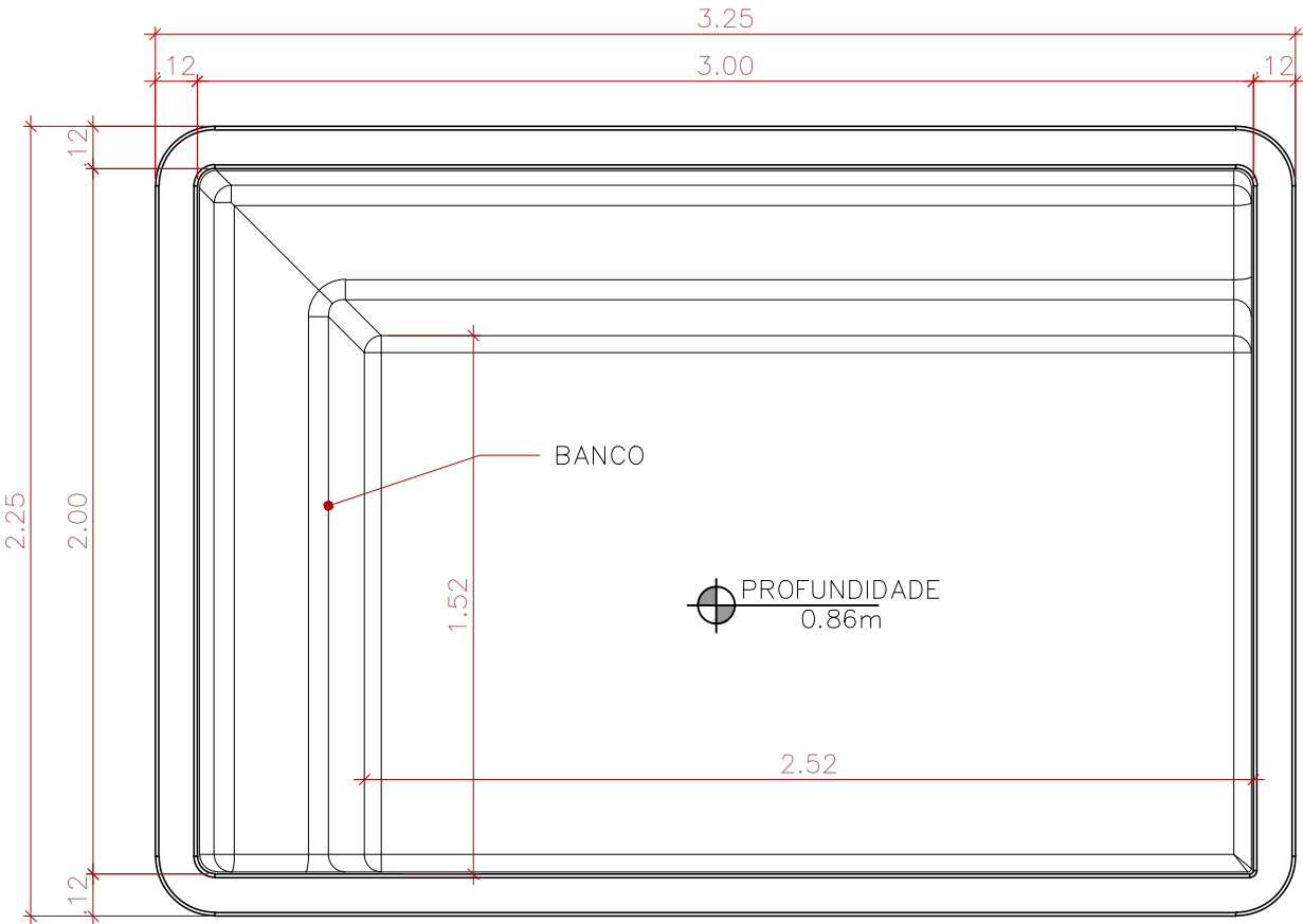
PLANTA BAIXA SEM ESCALA
