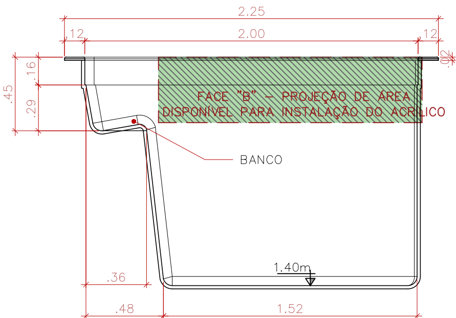
CORTE TRANSVERSAL SEM ESCALA
