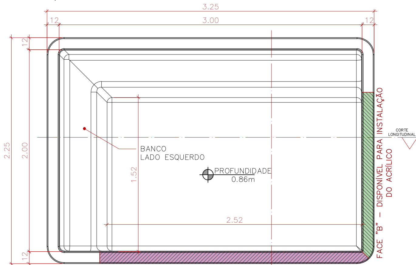
PLANTA BAIXA SEM ESCALA
