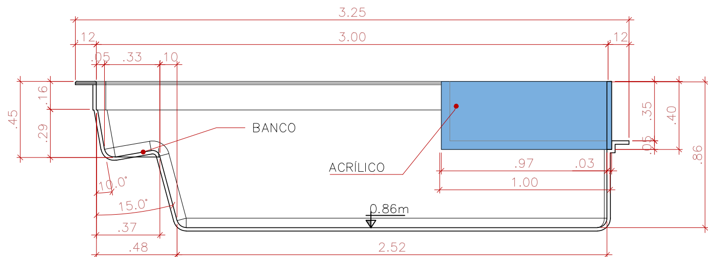
CORTE LONGITUDINAL SEM ESCALA
