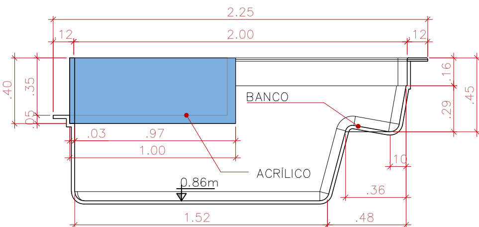
CORTE TRANSVERSAL SEM ESCALA
