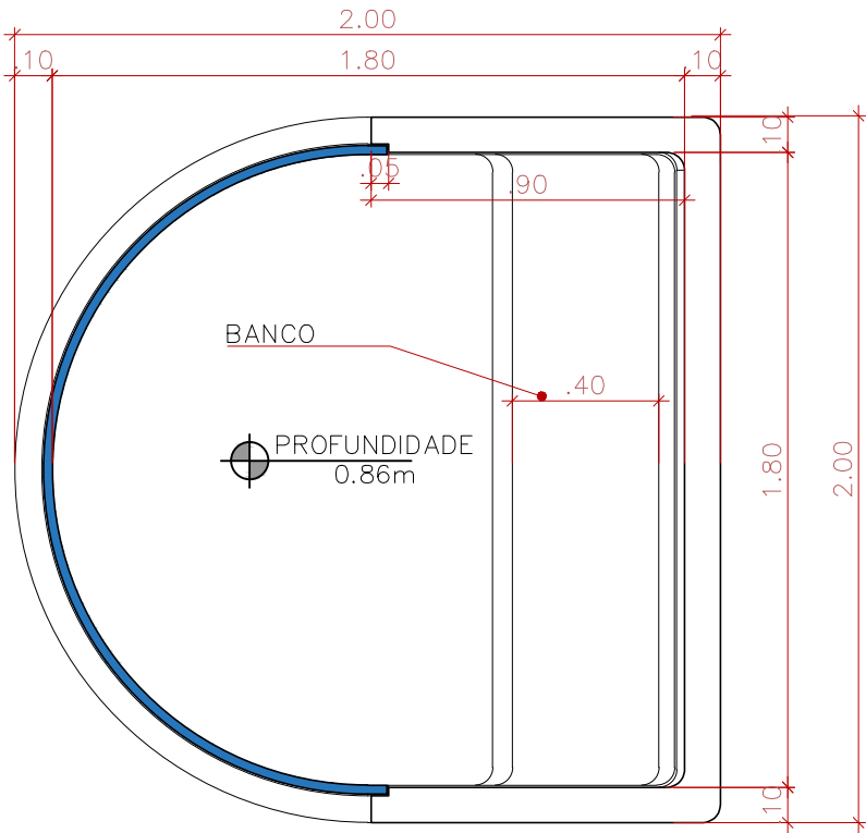
PLANTA BAIXA SEM ESCALA
