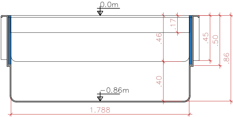
CORTE LONGITUDINAL SEM ESCALA
