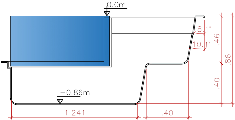
CORTE TRANSVERSAL SEM ESCALA
