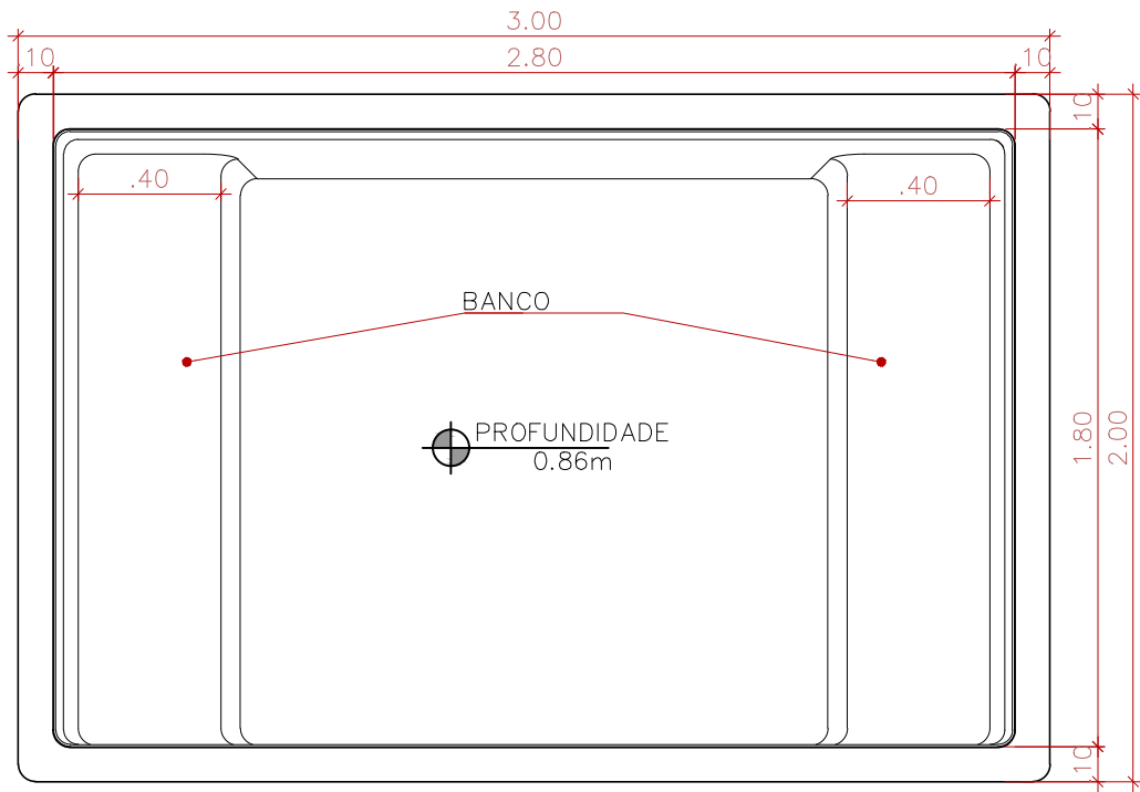
PLANTA BAIXA SEM ESCALA
