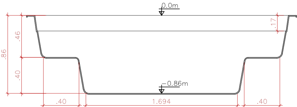
CORTE LONGITUDINAL SEM ESCALA
