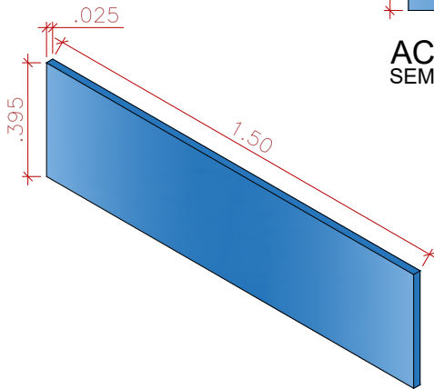
ACRÍLICO PERSPECTIVA SEM ESCALA
