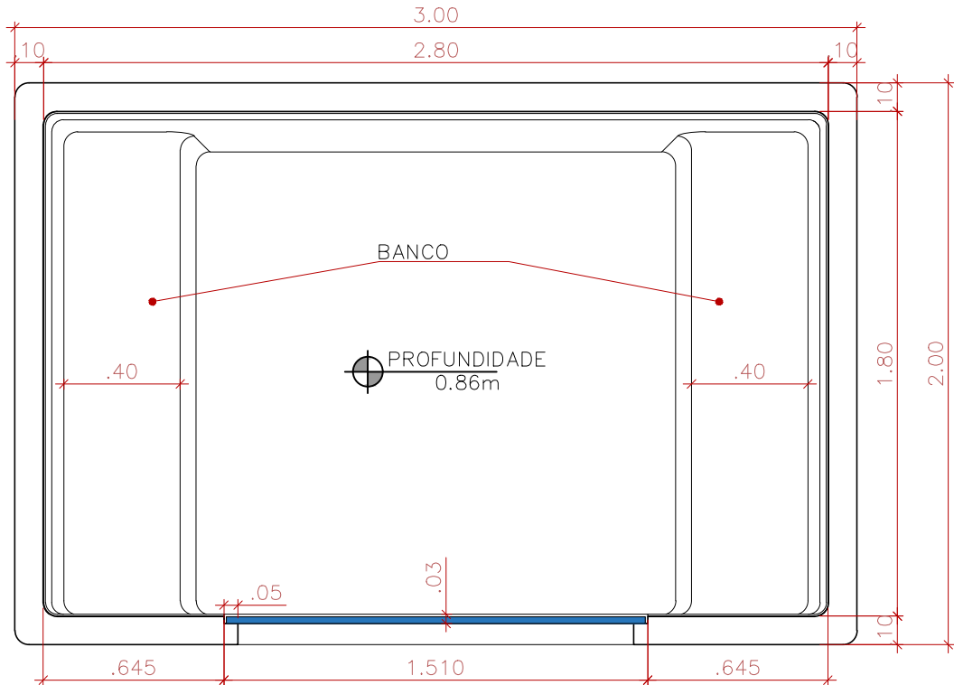
PLANTA BAIXA SEM ESCALA
