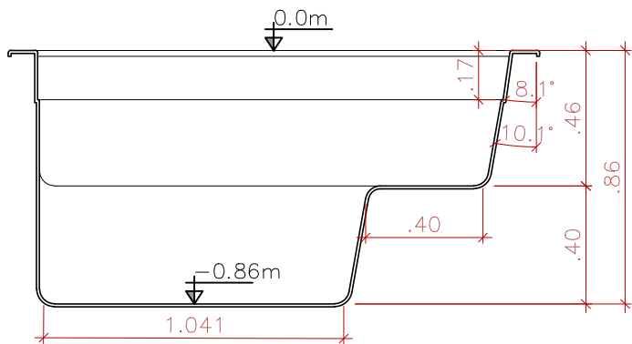
CORTE TRANSVERSAL SEM ESCALA
