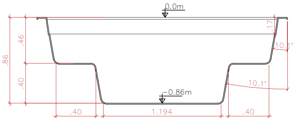
CORTE LONGITUDINAL SEM ESCALA
