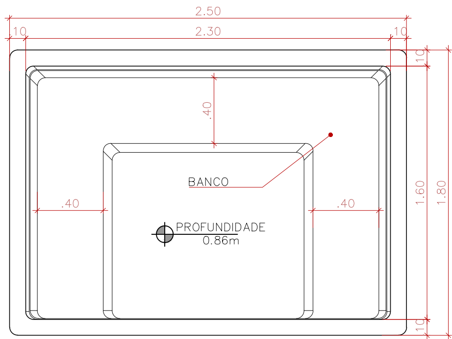
PLANTA BAIXA SEM ESCALA
