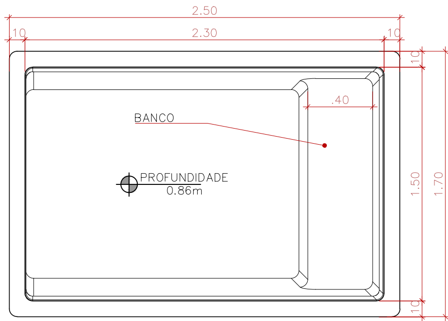
PLANTA BAIXA SEM ESCALA
