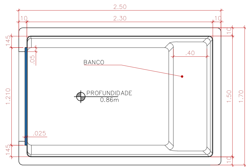
PLANTA BAIXA SEM ESCALA
