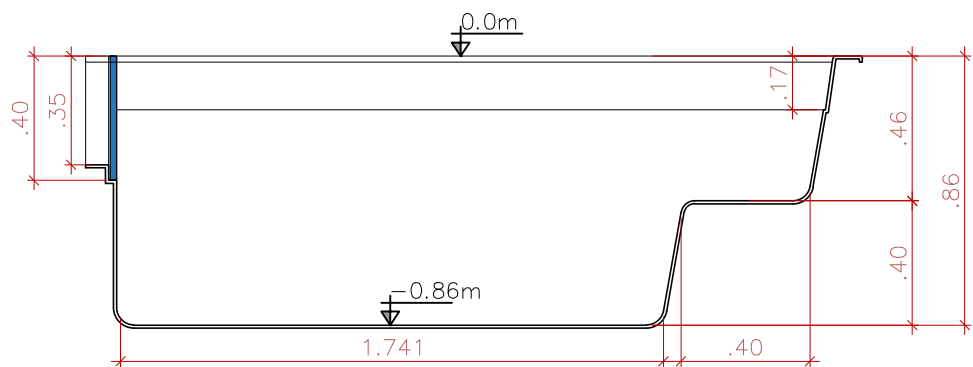
CORTE LONGITUDINAL SEM ESCALA
