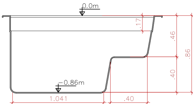
CORTE TRANSVERSAL SEM ESCALA
