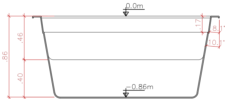
CORTE LONGITUDINAL SEM ESCALA
