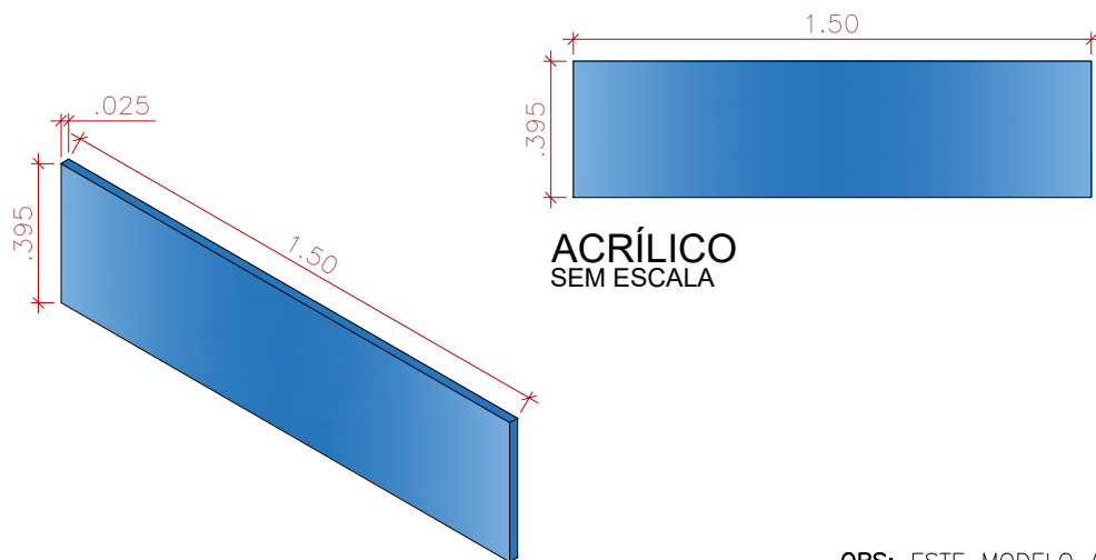
ACRÍLICO PERSPECTIVA SEM ESCALA
