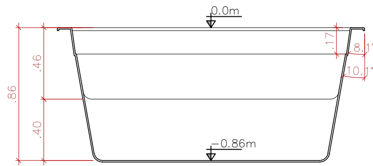
CORTE LONGITUDINAL SEM ESCALA
