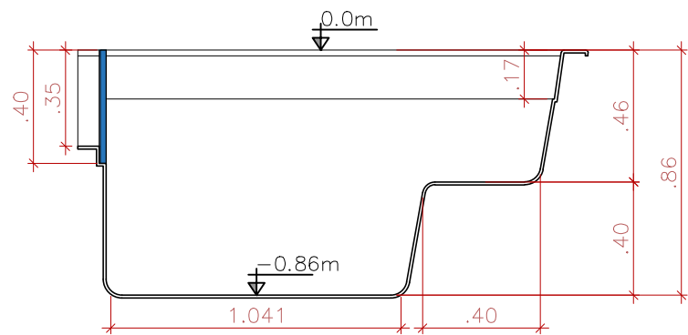
CORTE TRANSVERSAL SEM ESCALA
