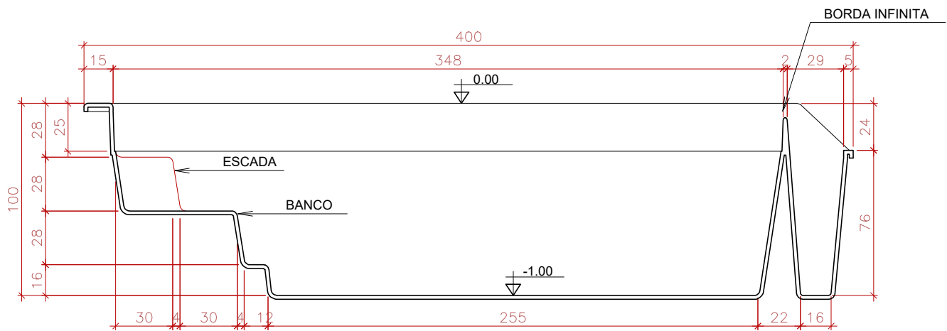
CORTE LONGITUDINAL SEM ESCALA
