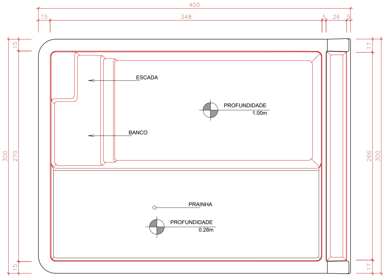
PLANTA BAIXA SEM ESCALA
