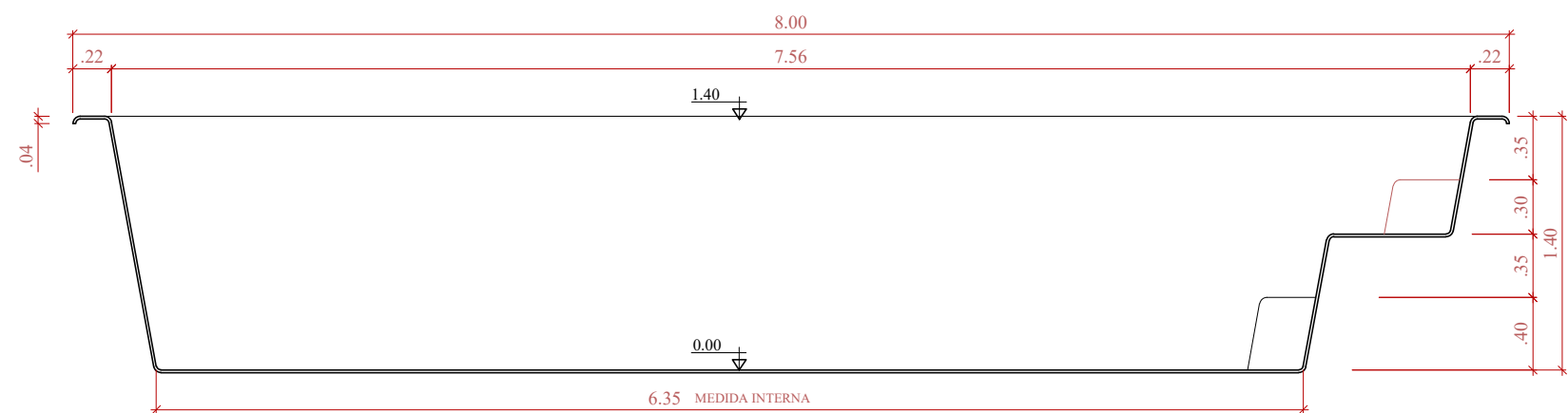
CORTE LONGITUDINAL SEM ESCALA
