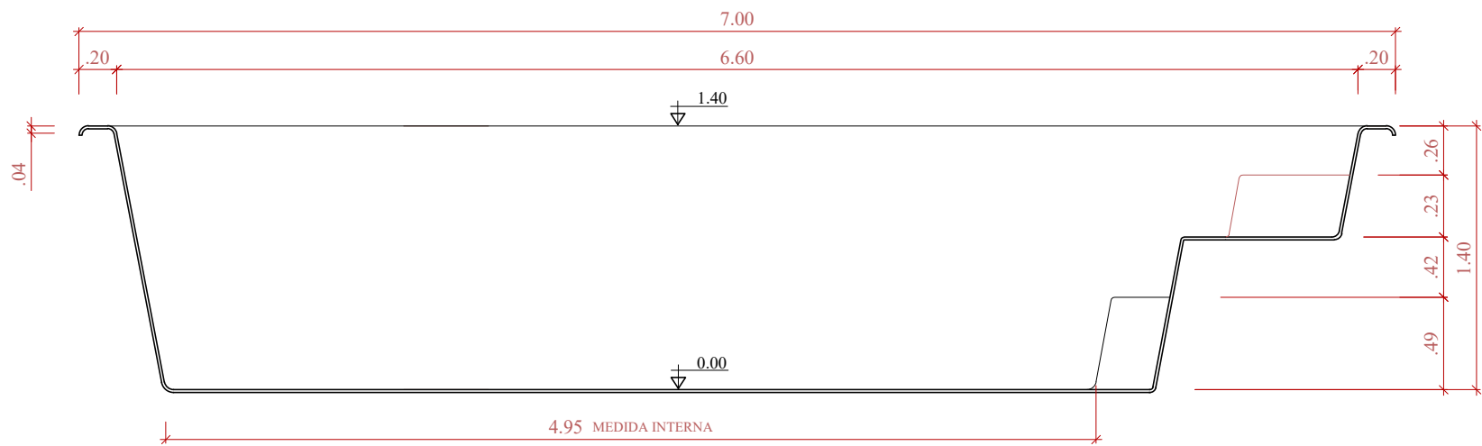
CORTE LONGITUDINAL SEM ESCALA
