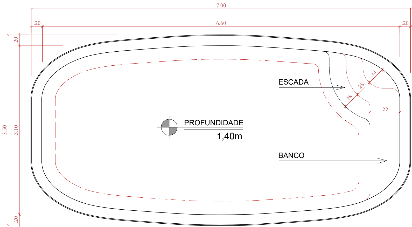
PLANTA SEM ESCALA
