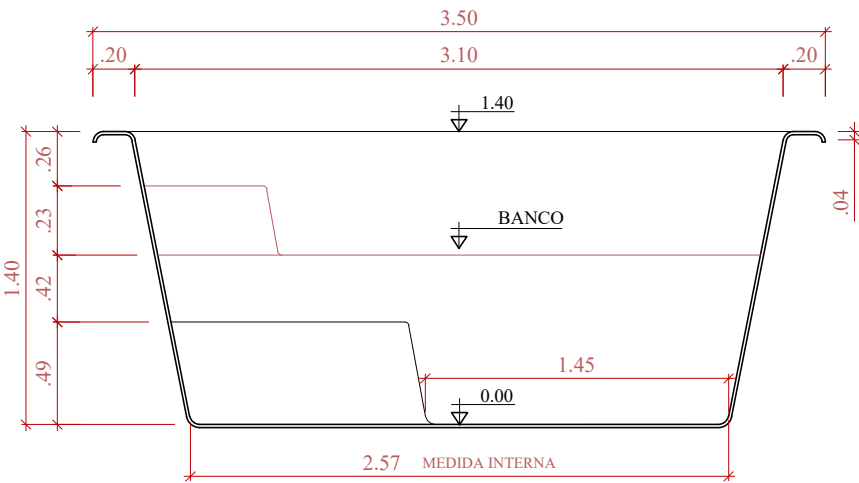
CORTE TRANSVERSAL SEM ESCALA
