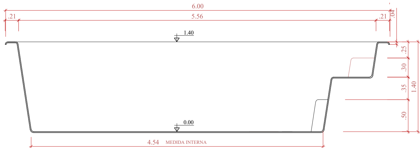
CORTE LONGITUDINAL SEM ESCALA
