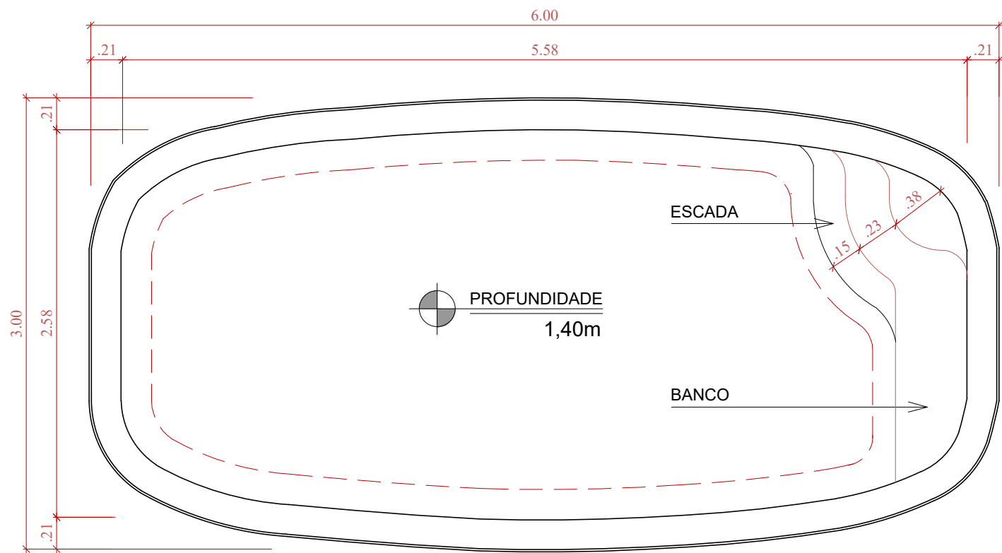
PLANTA SEM ESCALA
