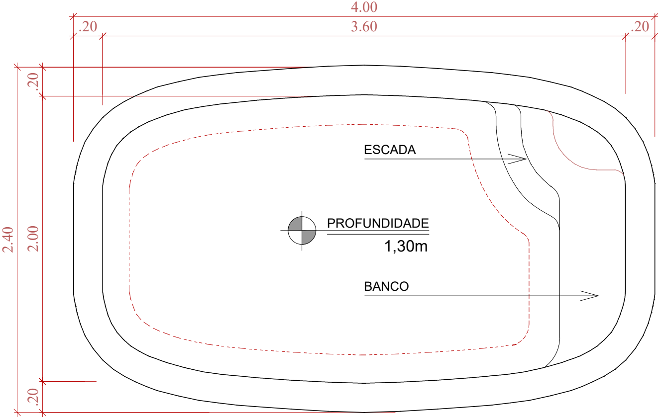
PLANTA SEM ESCALA
