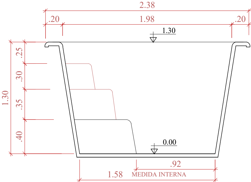
CORTE LONGITUDINAL SEM ESCALA
