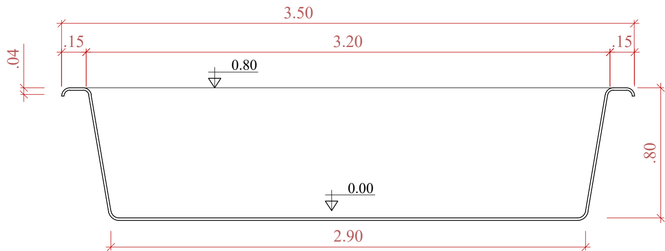
CORTE LONGITUDINAL SEM ESCALA
