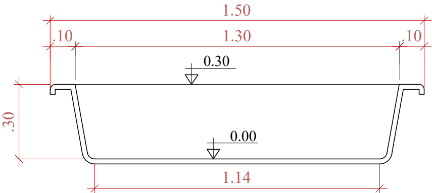
CORTE TRANSVERSAL SEM ESCALA
