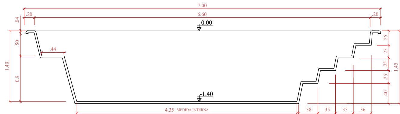
CORTE LONGITUDINAL SEM ESCALA
