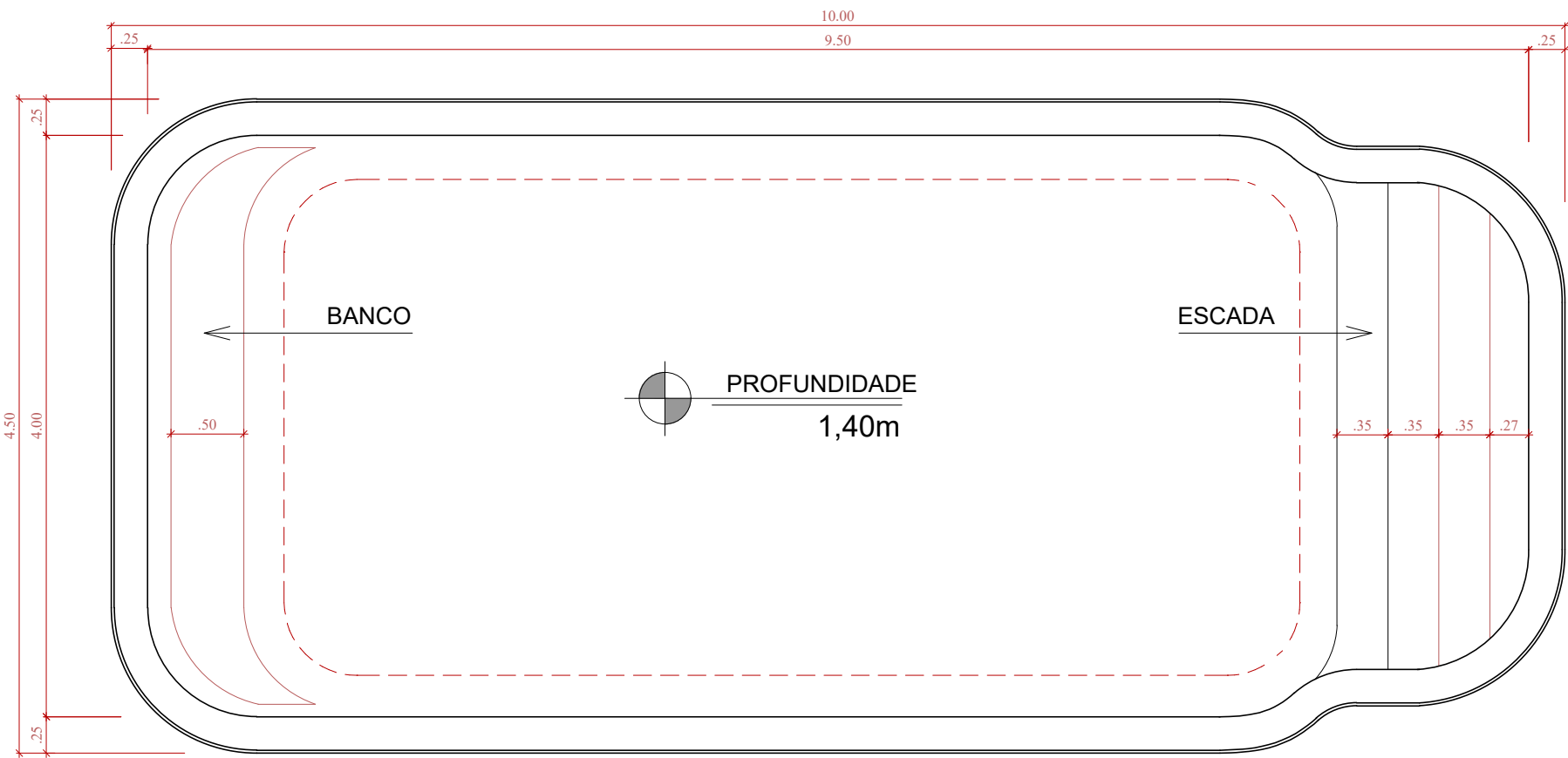
PLANTA SEM ESCALA
