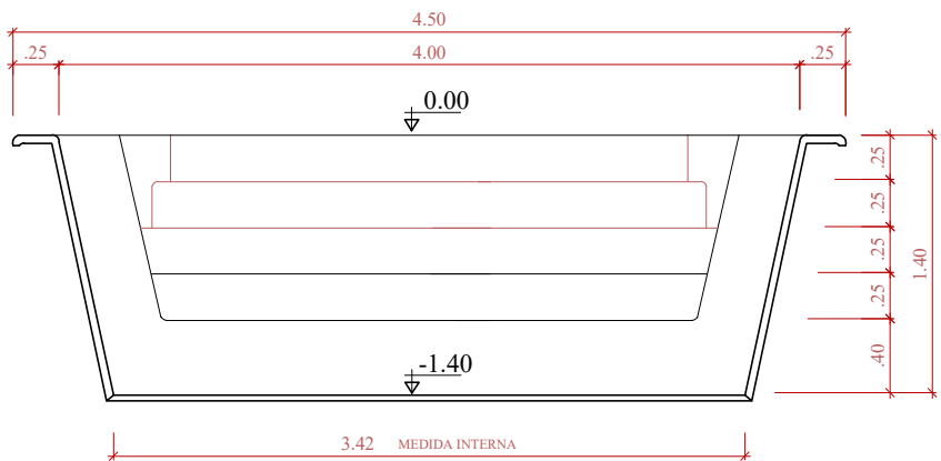
CORTE TRANSVERSAL SEM ESCALA
