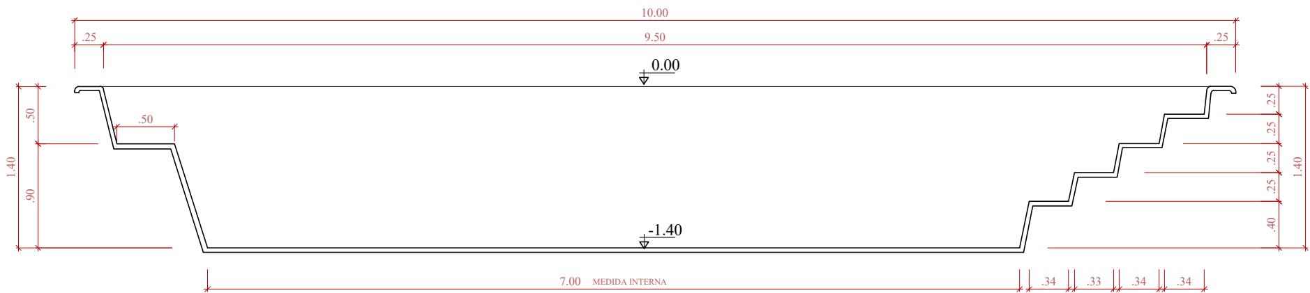
CORTE LONGITUDINAL SEM ESCALA
