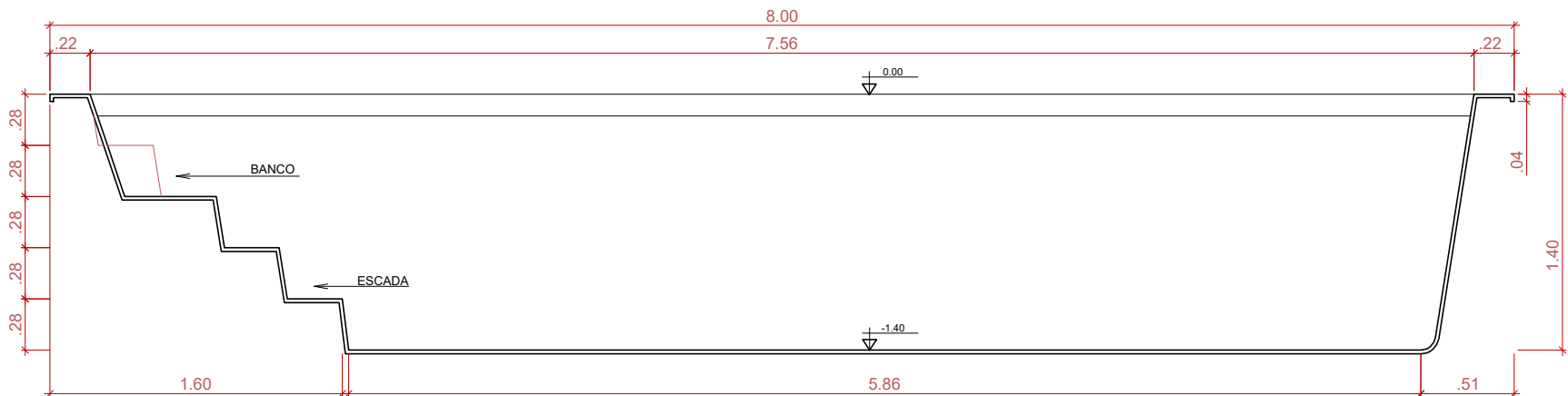
CORTE LONGITUDINAL SEM ESCALA
