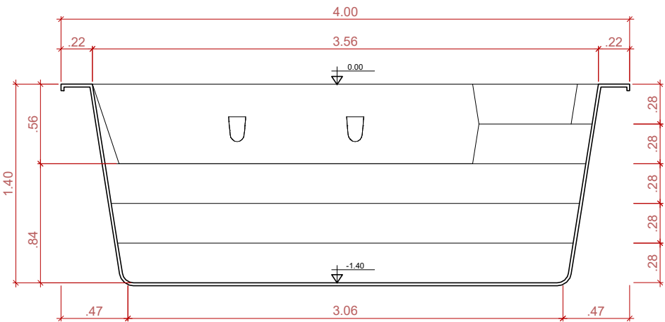
CORTE TRANSVERSAL SEM ESCALA
