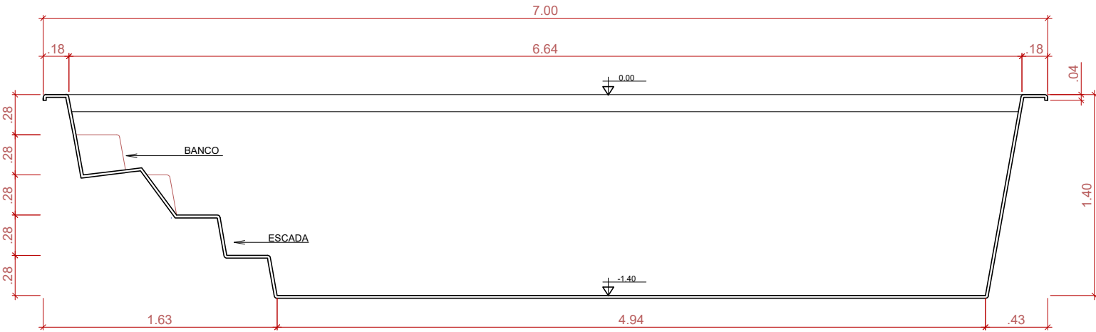
CORTE LONGITUDINAL SEM ESCALA
