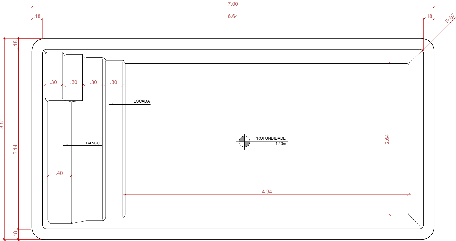
PLANTA BAIXA SEM ESCALA
