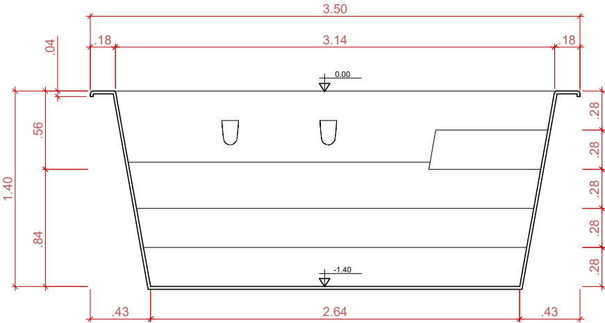
CORTE TRANSVERSAL SEM ESCALA
