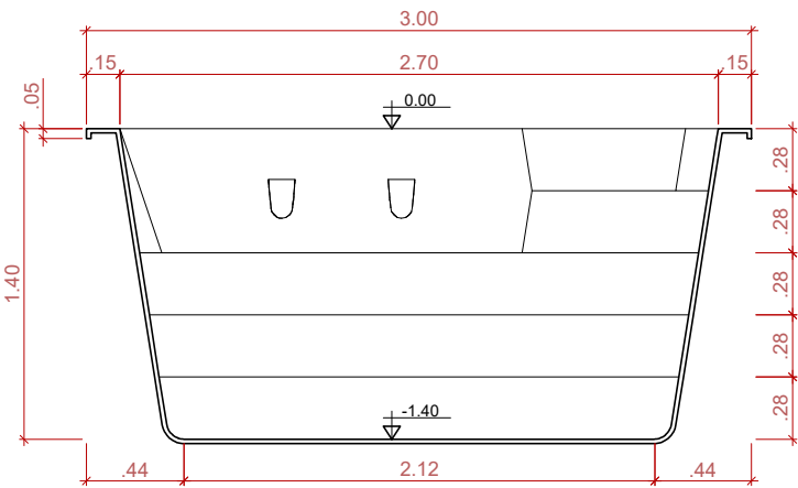
CORTE TRANSVERSAL SEM ESCALA
