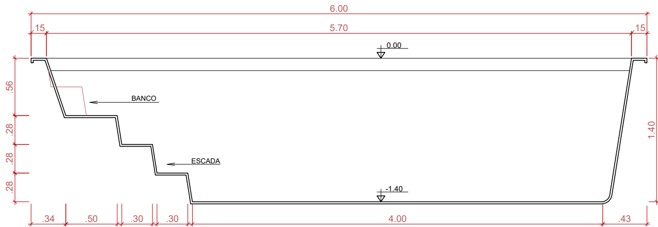
CORTE LONGITUDINAL SEM ESCALA
