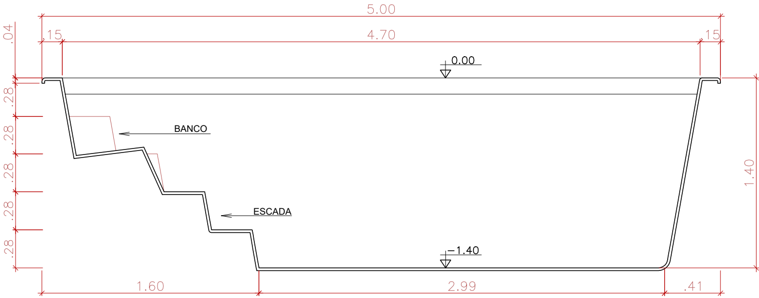
CORTE LONGITUDINAL SEM ESCALA
