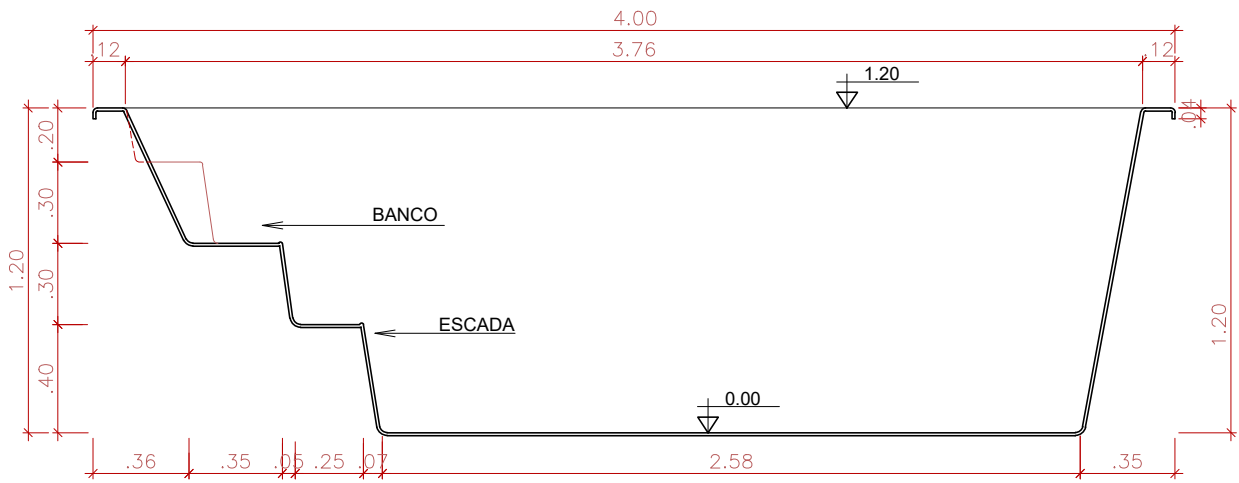
CORTE LONGITUDINAL SEM ESCALA
