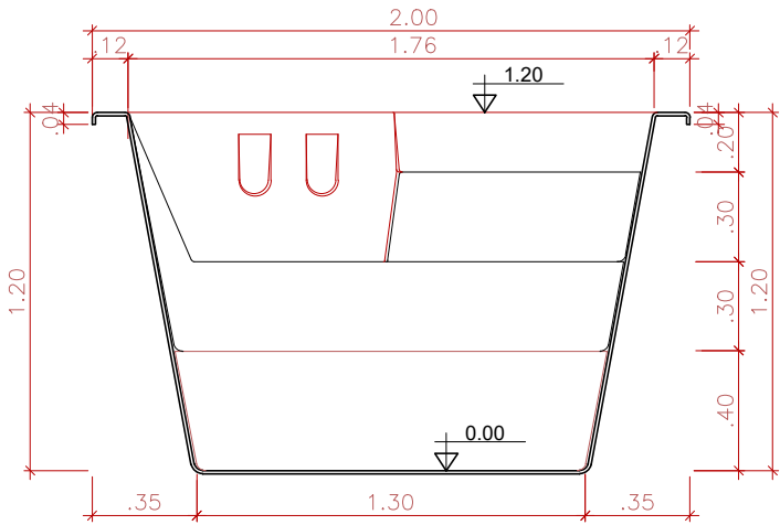
CORTE TRANSVERSAL SEM ESCALA
