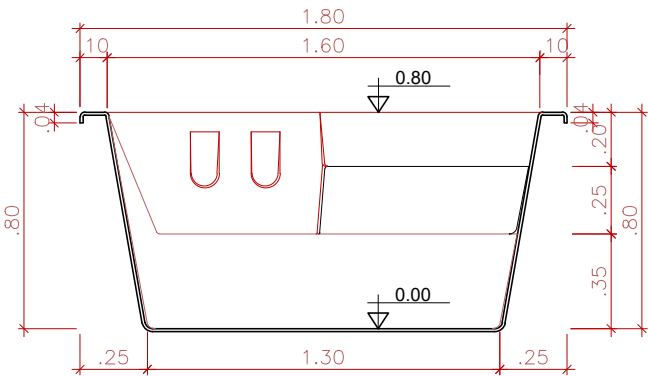
CORTE TRANSVERSAL SEM ESCALA
