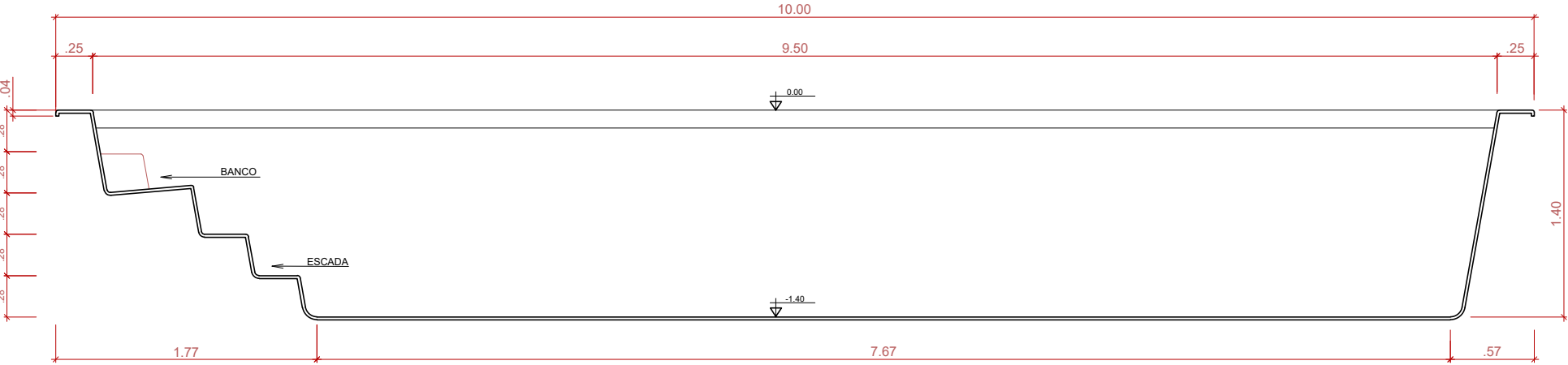
CORTE LONGITUDINAL SEM ESCALA
