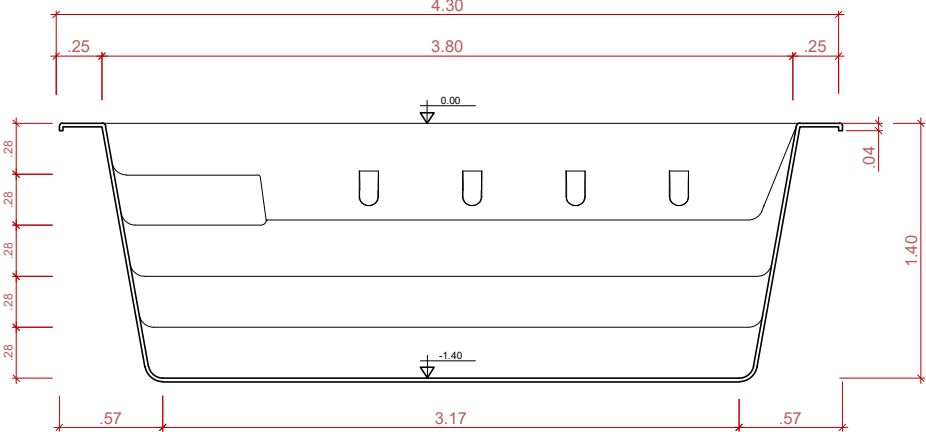
CORTE TRANSVERSAL SEM ESCALA
