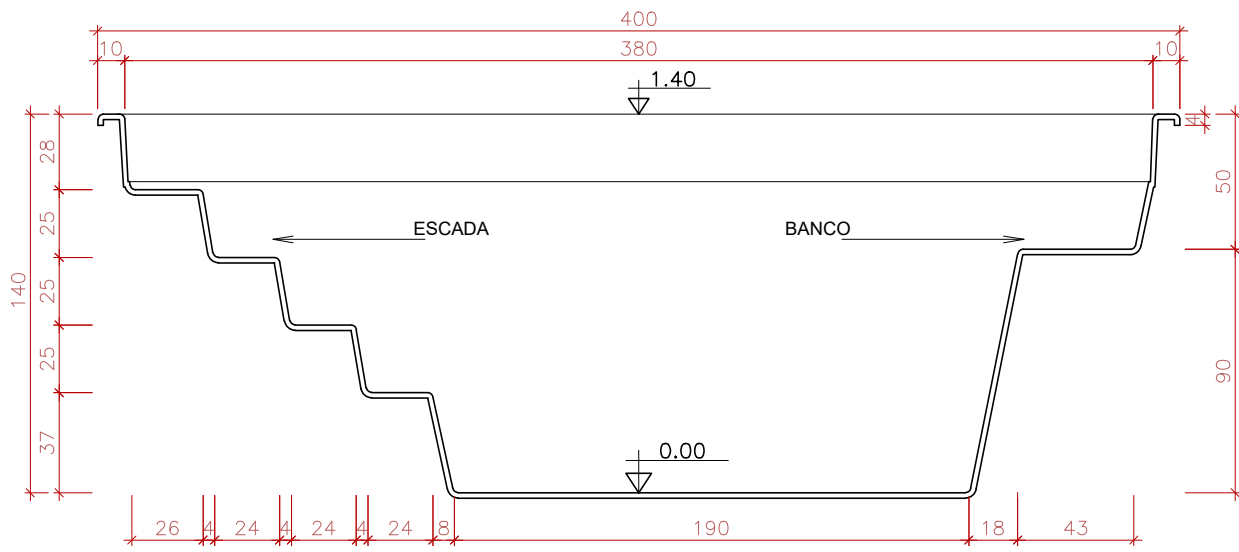
CORTE LONGITUDINAL SEM ESCALA
