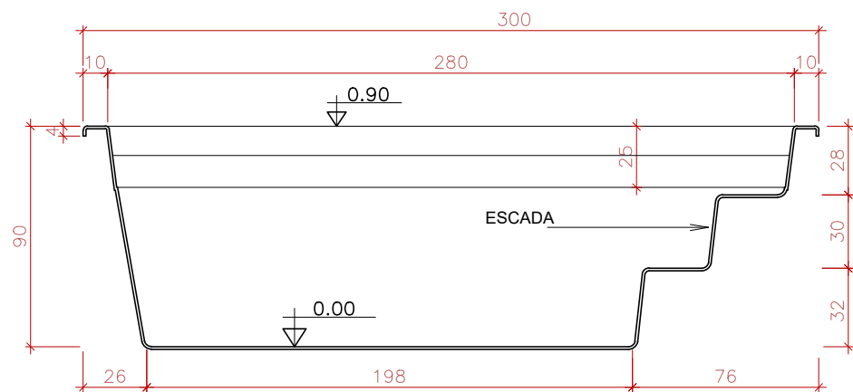
CORTE LONGITUDINAL SEM ESCALA
