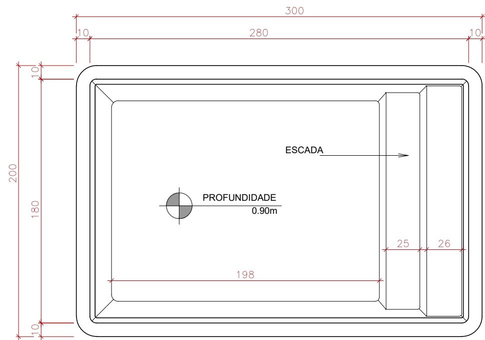
PLANTA BAIXA SEM ESCALA
