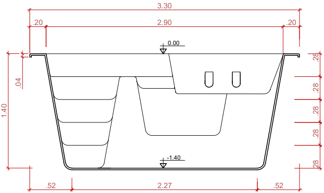
CORTE TRANSVERSAL SEM ESCALA
