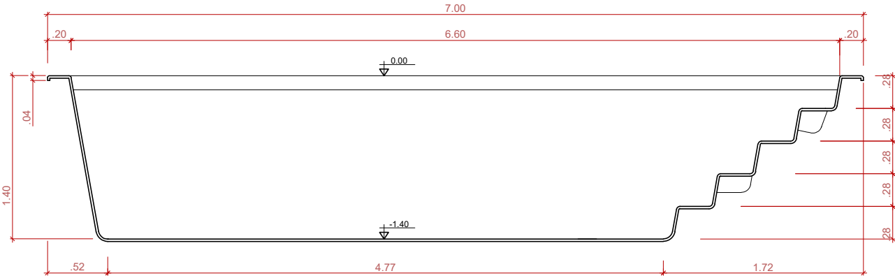
CORTE LONGITUDINAL SEM ESCALA
